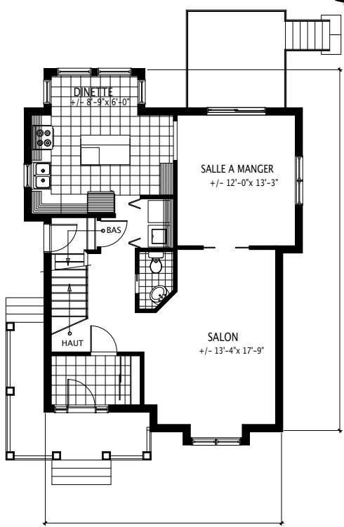
Plan du rez-de-chaussée Sup. 863 pi. ca.
