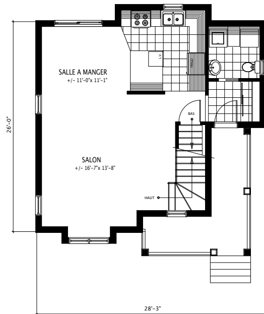
Plan du rez-de-chaussée Sup. 653pi. ca.
