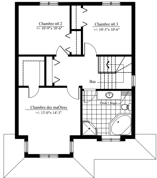
Plan du rez-de-chaussée Sup. 740 pi. ca.
