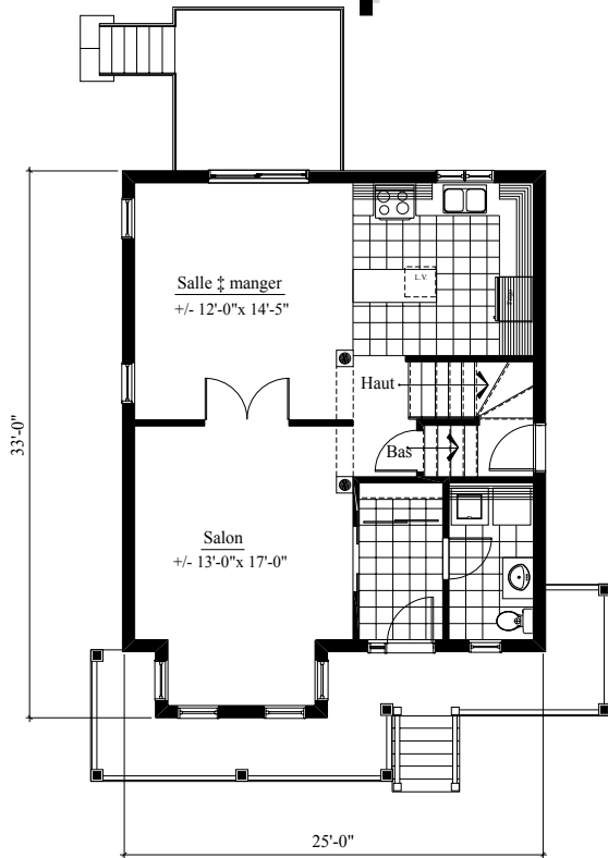
Plan de l'Étage Sup. 740 pi. ca.
