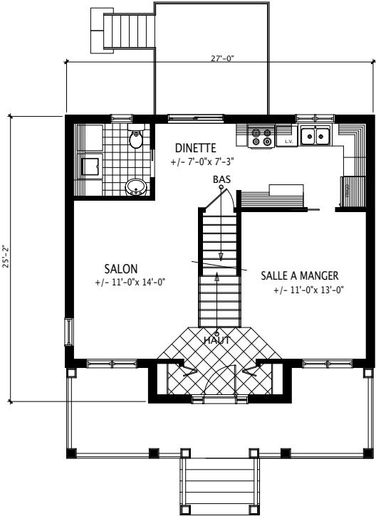
Plan du rez-de-chaussée Sup. 633 pi. ca.
