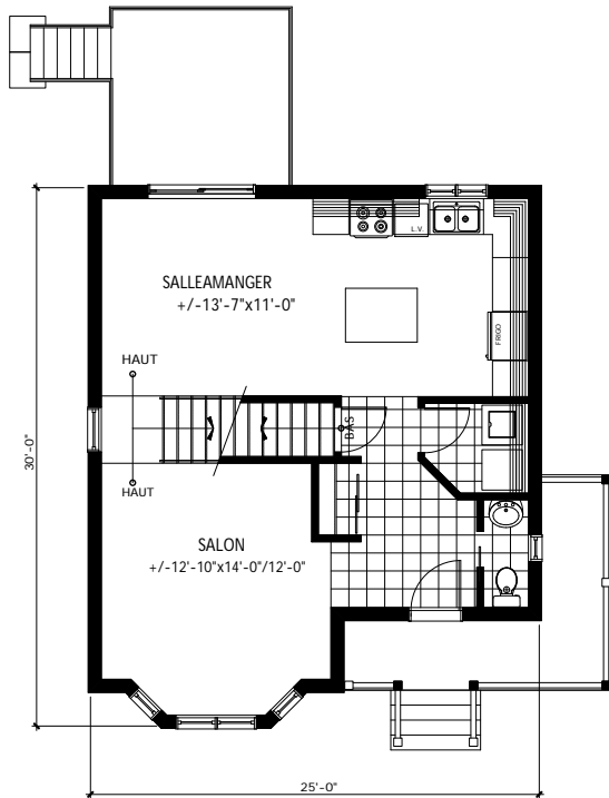
Plan du rez-de-chaussée Sup. 670 pi. ca.
