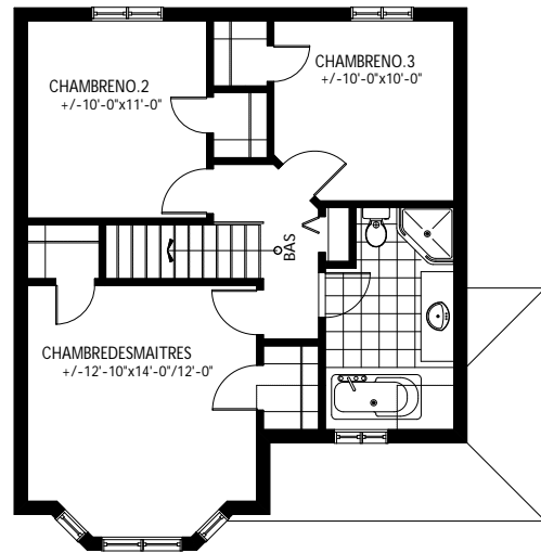
Plan de l'Étage Sup. 670 pi. ca.
