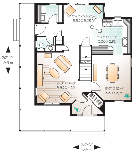
Rez-de-chaussée: 802 pi 2 (72,2 m 2 )
